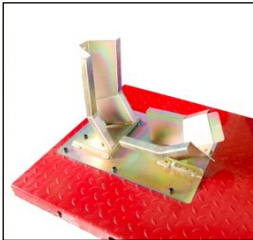
Mordaza delantera ajustable para fijar la motocicleta
